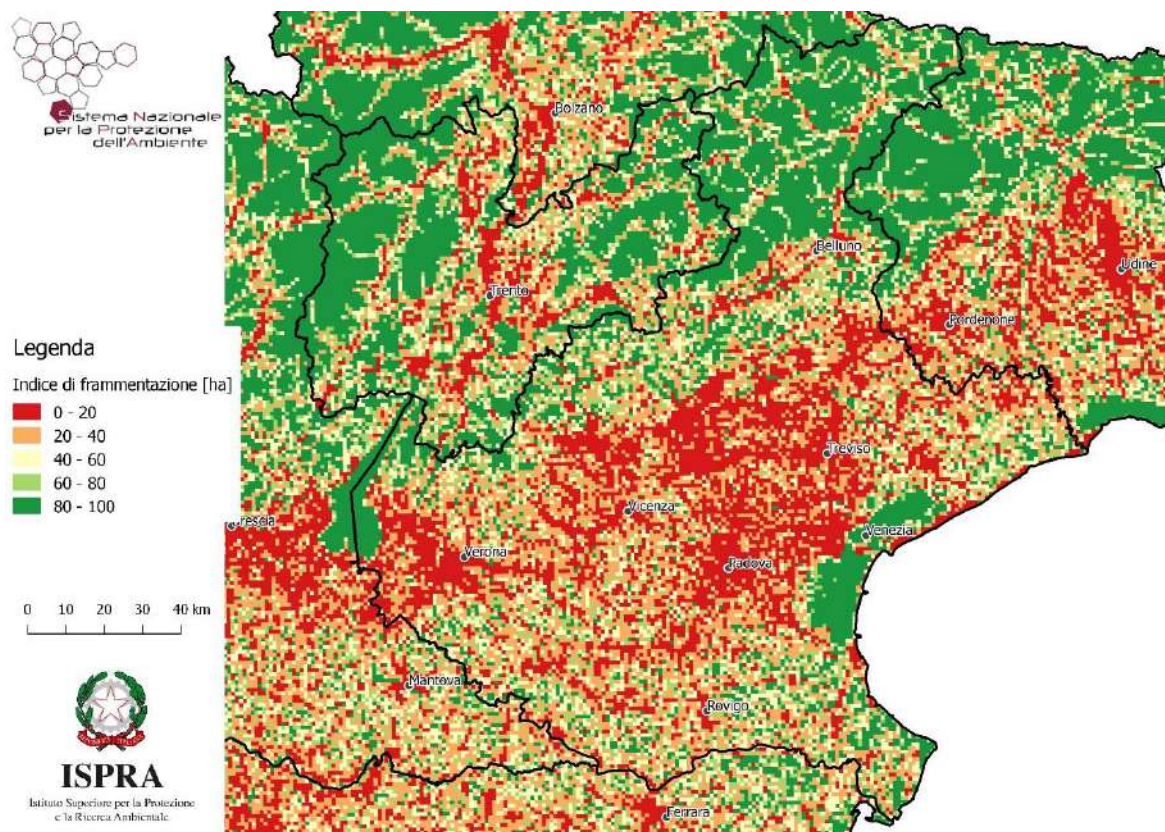
Figura 67 - Indice di frammentazione ( mesh size ) al 2016
