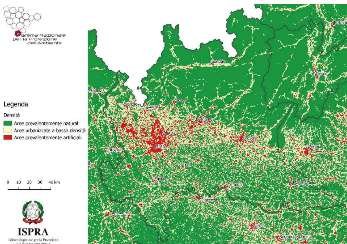
Figura 44 - Densità del consumo di suolo (1. Aree prevalentemente naturali/artificiale assente o rado; 2. Aree a media/bassa densità di copertura artificiale; 3. Aree prevalentemente artificiali /artificiale compatto)
