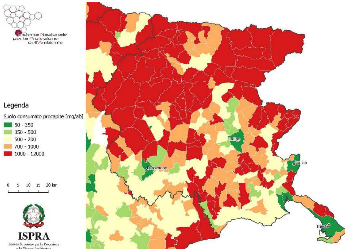
Figura 73 - Consumo di suolo procapite a livello comunale (m 2 /ab 2016)
