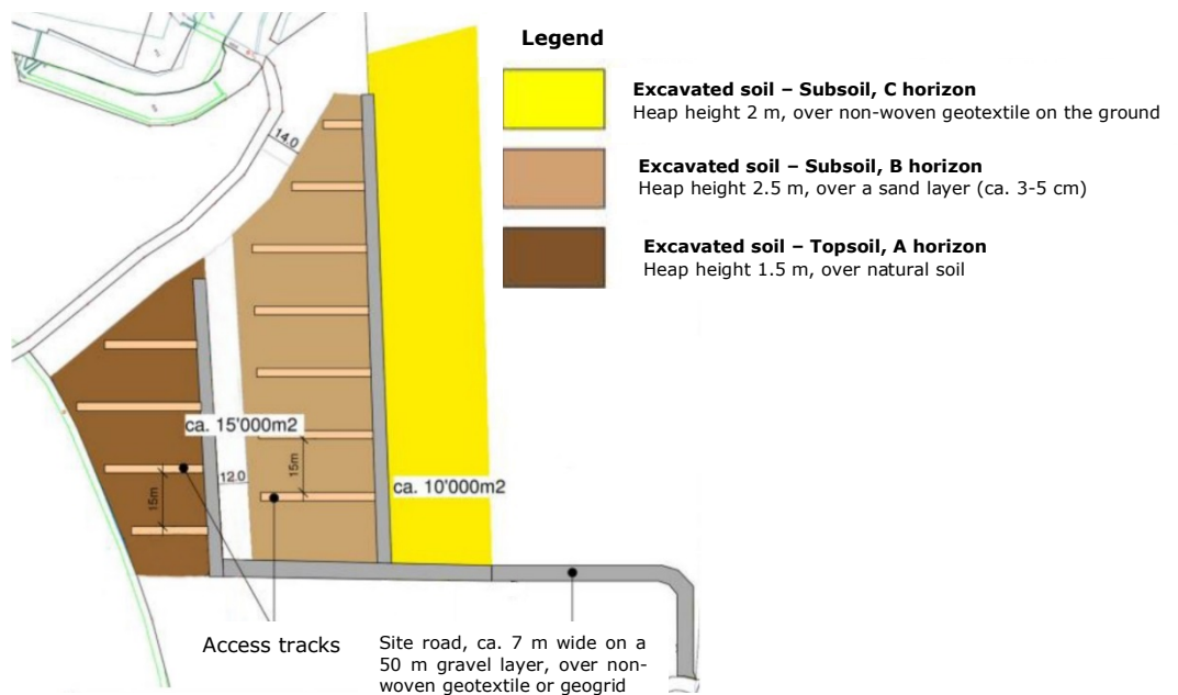
Figure 19. Example of a plan of soil storage areas (source: Suolo e cantieri. Stato della tecnica e della prassi UFAM 2015, mod.)
