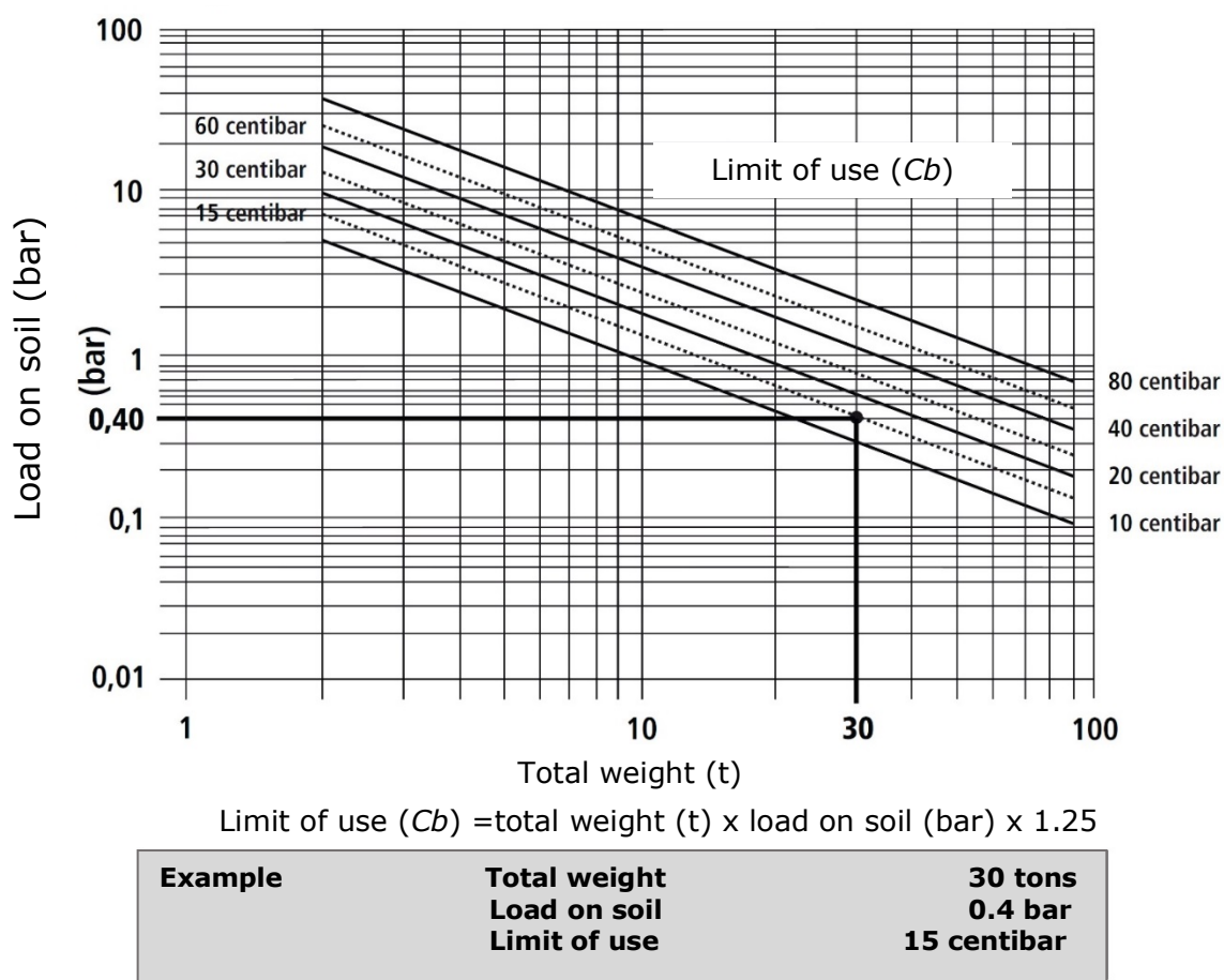
Figure 16. Nomogram for the limit of use of machinery at construction sites (source: Costruire proteggendo il suolo. Guida all'ambiente n. 10. Ufficio federale dell'ambiente, delle foreste e del paesaggio, UFAFP, 2001 )
